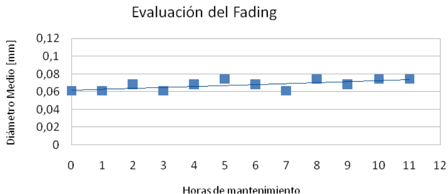
Gráfico 1. Diámetro medio del grano en función de las horas de mantenimiento del líquido a 950 +/- 10 °C
