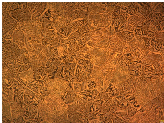
Fig. 3 – Estructura de latón después de estar 12 horas en estado líquido a 950°C
